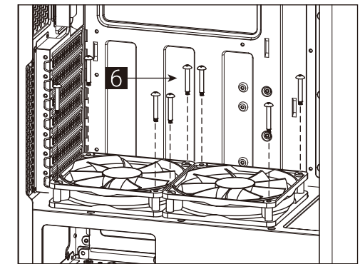
(7c) Install VGA Fan
